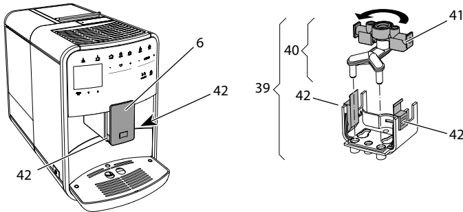
Abb. 22: Einlauf drehen
