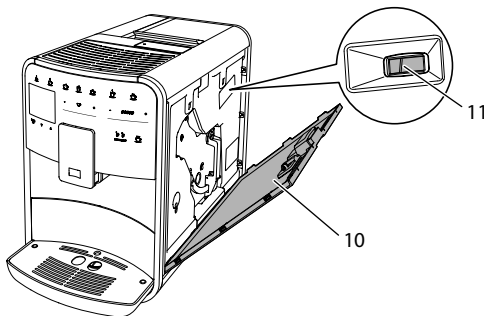
Abb. 21: Mahlgrad einstellen
