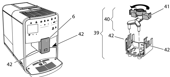
Fig. 22: Rotazione del tubo di mandata latte
