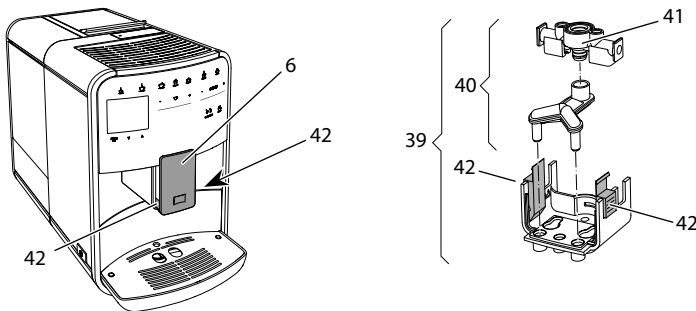
Abb. 24: Milcheinheit ausbauen
